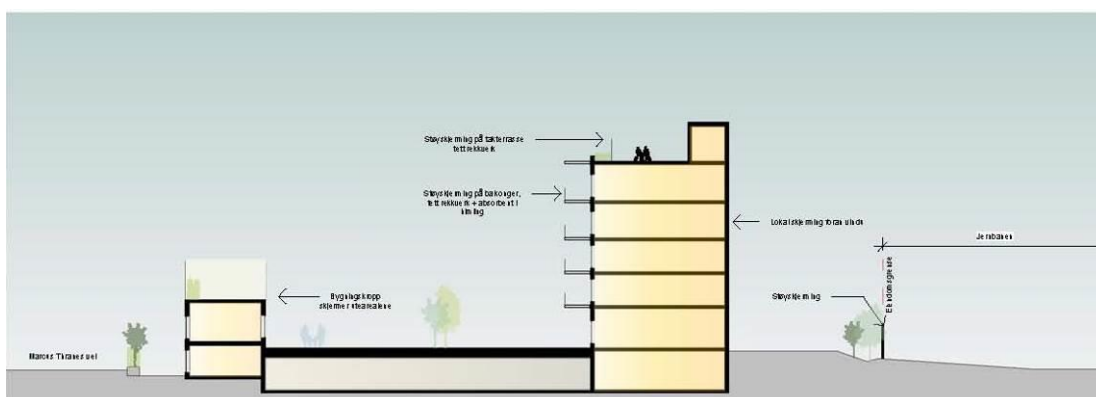
Prinsippsnitt C-C som viser støyskjerming, ill: Arcasa Arkitekter as
