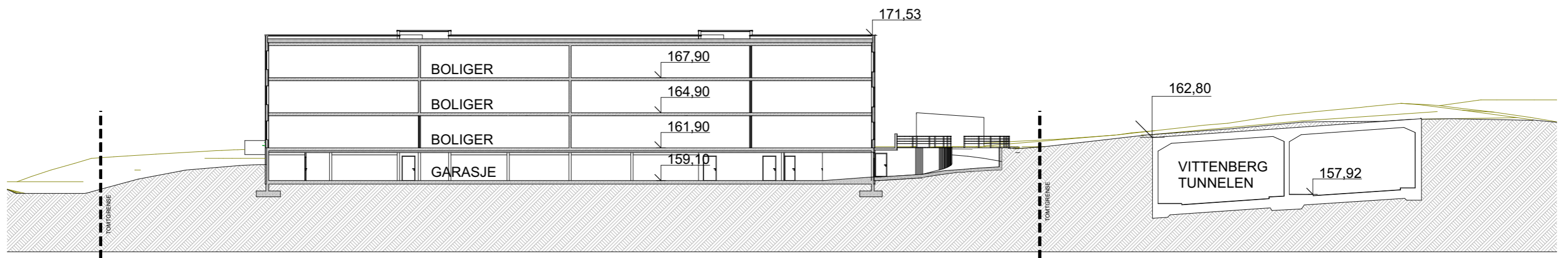
1:350 Snitt B
