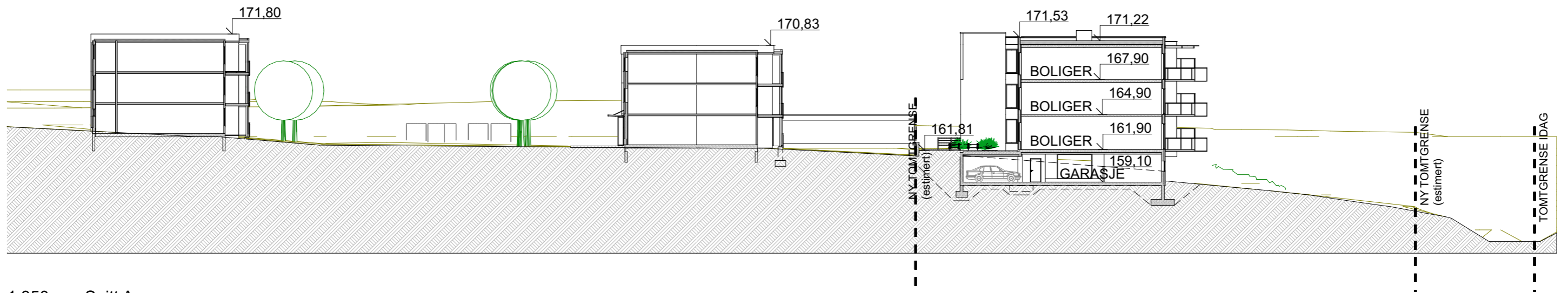
1:350 Snitt A
