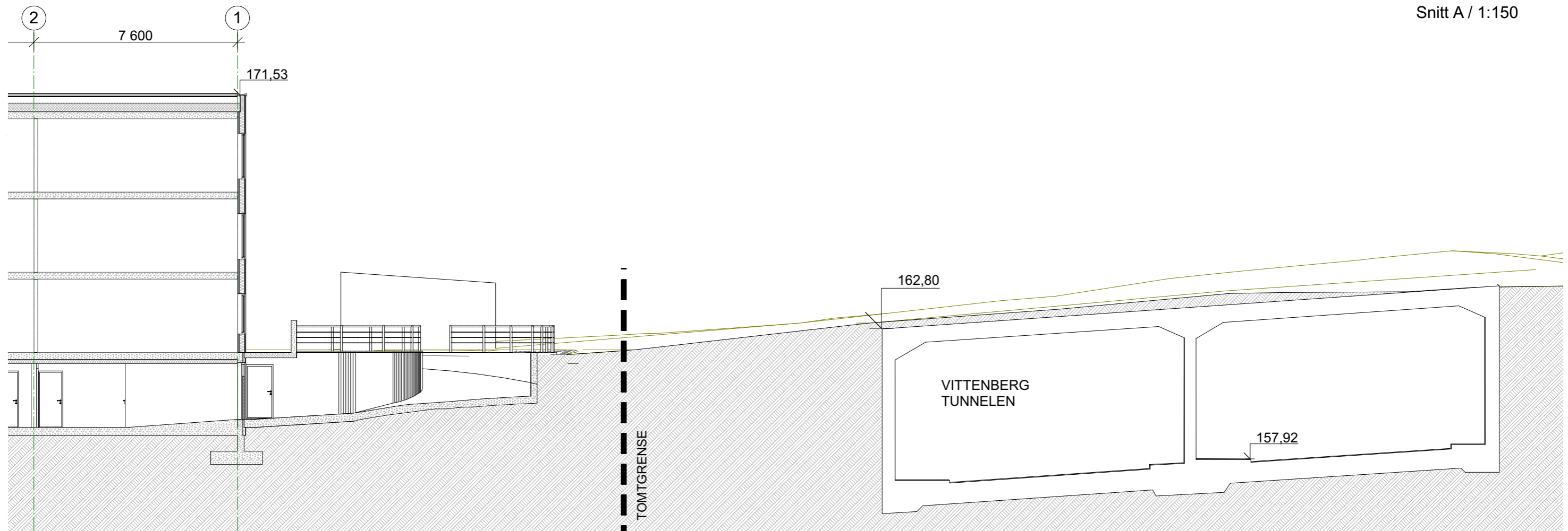
Snitt B / 1:150
