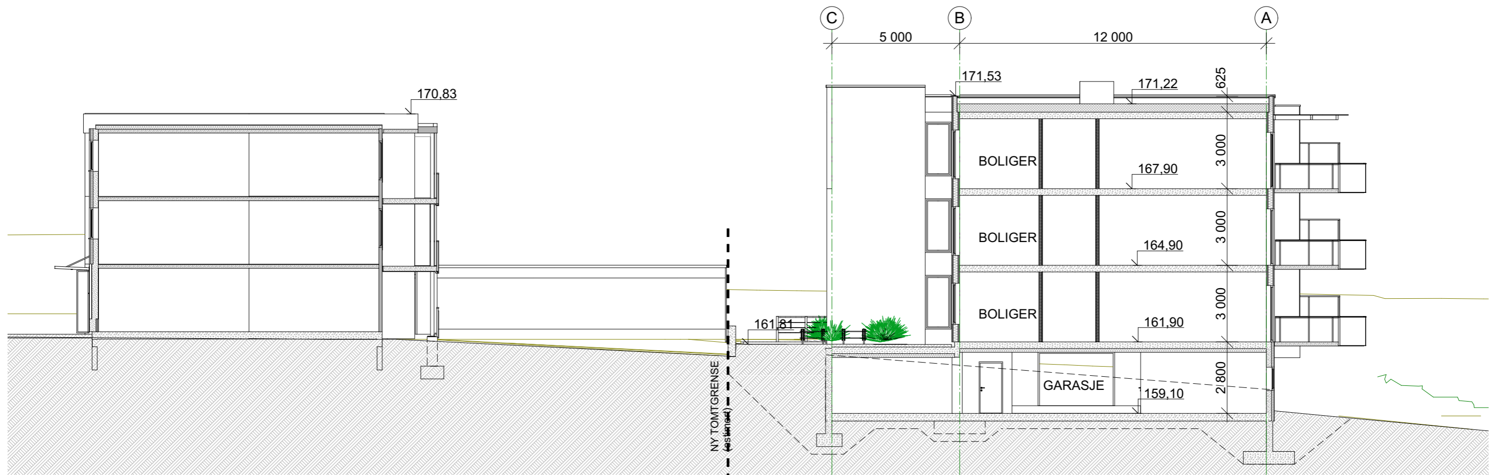
Snitt A / 1:150
