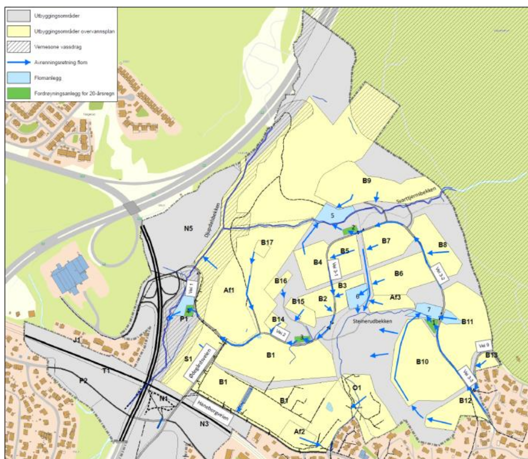
Figur 2 Flomplan for Lørenskog Stasjonsby ved Q200+20% (COWI, 2016)
