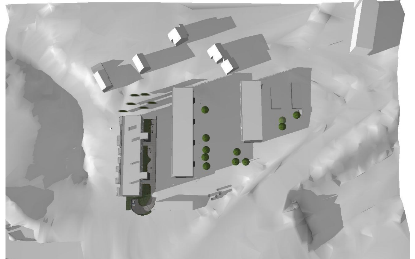
solstudie 21 mars kl 18
